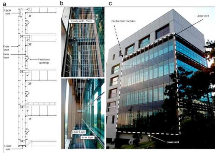
شكل (9) تفاصيل لواجهة بنظام الجلد المزدوج
