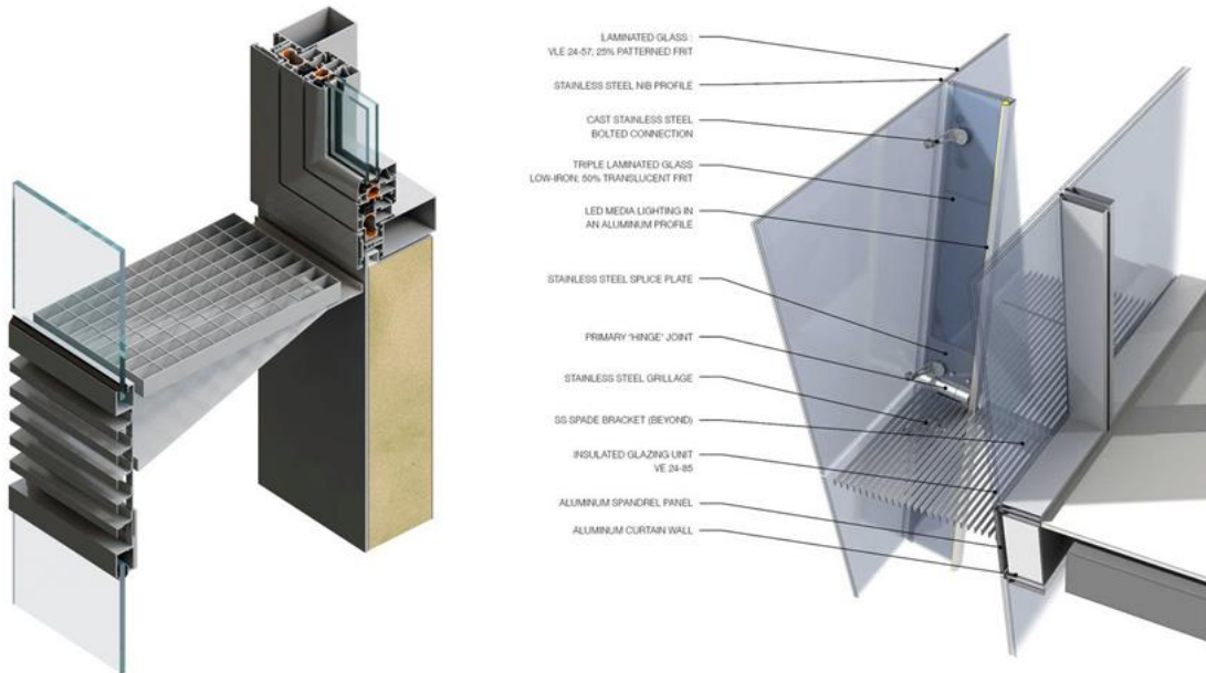
شكل (8) تفاصيل داخلية لنظام الجلد المزدوج
