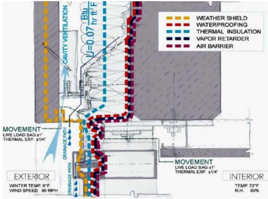
شكل (2) قطاع يوضح كل وظيفة من خلال خط على رسومات الواجهة
