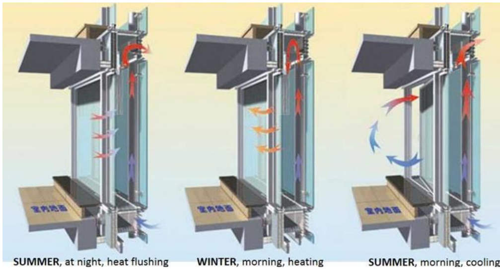
شكل (6) كيفية عمل واجهة الجلد المزدوج صيفا وشتانا
